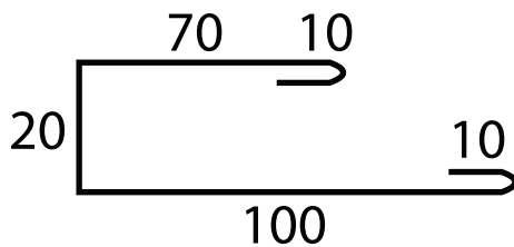
Door Side Flashing
